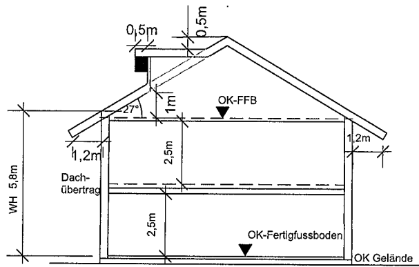
Giebelgaube / Schleppgaube ab 27°
