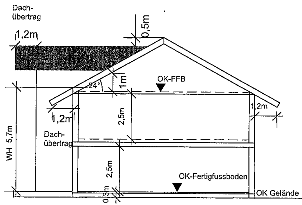
Quergiebel / Standgiebel ab 24°
